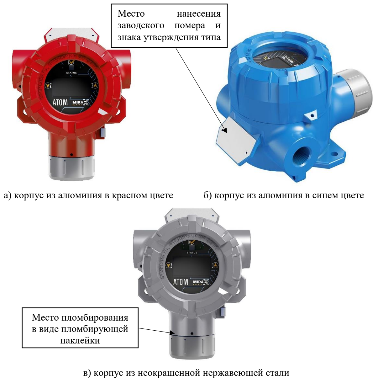
Рисунок 1 – Общий вид газоанализаторов стационарных АТОМ, а также место и метод пломбирования от несанкционированного доступа
